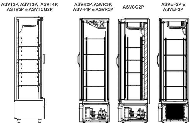
Figura 12: Prateleiras dos produtos da linha Auto Serviço
