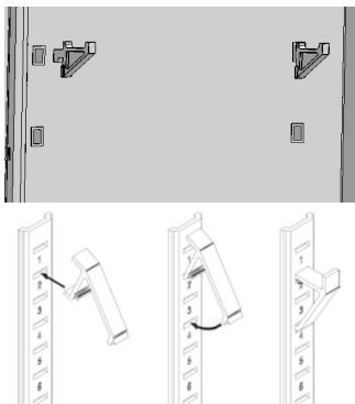
Figura 10: Fixação dos suportes das prateleiras
