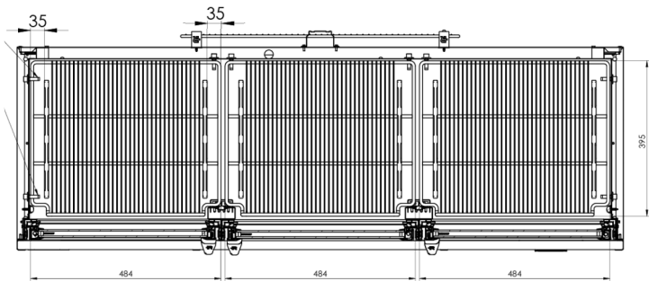
Figura 10: Fixação dos suportes das prateleiras
