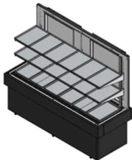
Figura 12: Colocação das bandejas no suporte
