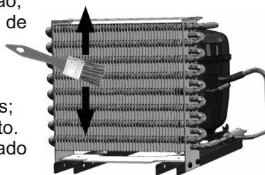
Figura 20: Limpando o condensador.
