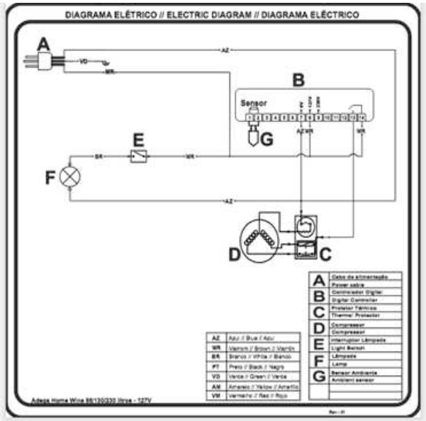
Figura 16: Diagrama eléctrico modelos AHW – 127V
