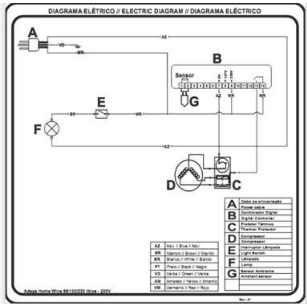
Figura 16: Diagrama eléctrico modelos AHW - 220V
