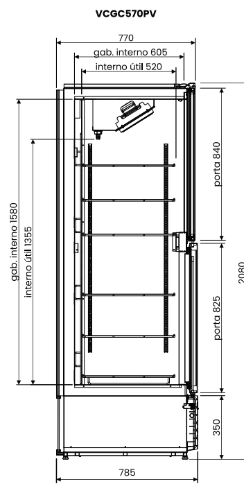
VISA COOLER GELA CANECAS 570L PORTA DE VIDRO
