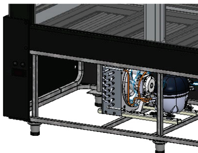
Figura 17: Unidade condensadora e controlador digital
