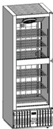
Figura 8: Colocação das grades (Arco virado para o fundo do gabinete)
