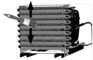
Figura 17: Limpando o condensador
