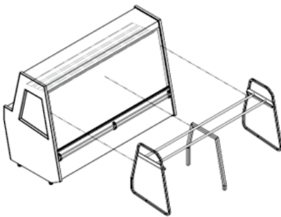
Figura 10: Gancheiras
