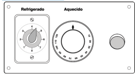
Figura 5: termostato mecânico para refrigeração e aquecimento.
