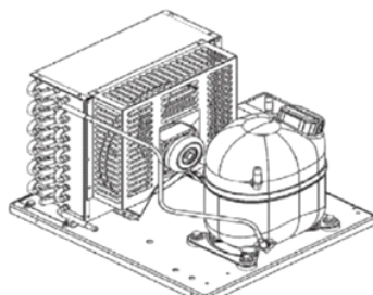
Figura 14: Unidade Condensadora
