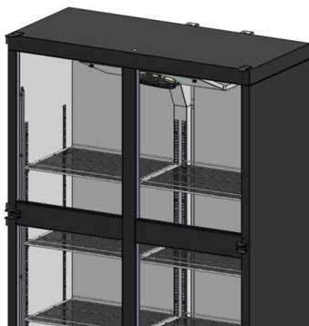
Figura 10: Colocação das prateleiras modelo 900.
