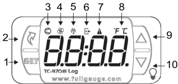
Figura 7: Controlador Digital TC 970E LOG
