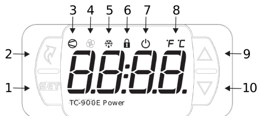
Figura 6: Controlador TC-900 POWER
