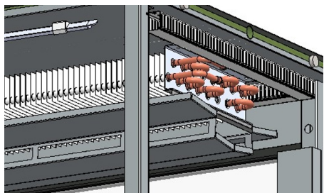
Figura 16: Evaporador Estático
