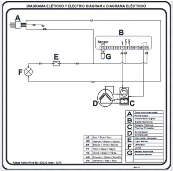
Figura 15: Diagrama elétrico modelos AHW – 127V
