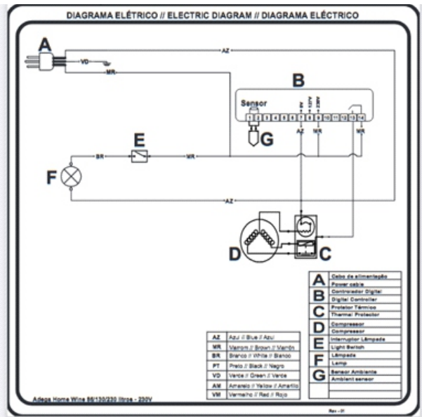
Figura 16: Diagrama elétrico modelos AHW - 220V
