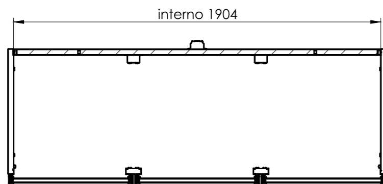
SEÇÃO B-B
