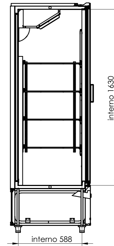
SEÇÃO A-A
