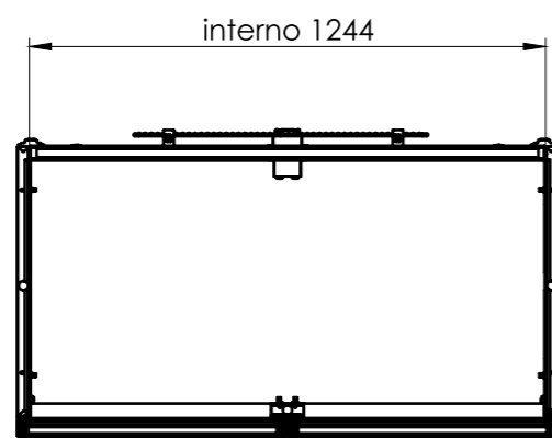
SEÇÃO B-B
