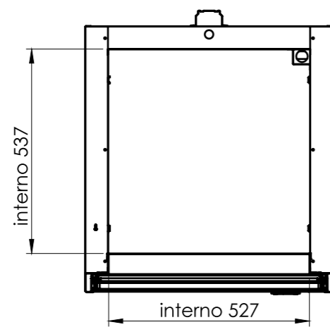
SEÇÃO B-B
