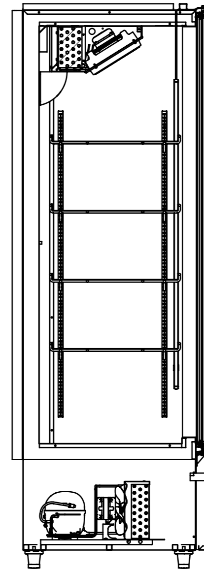
SEÇÃO A-A
