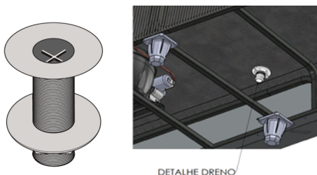
Figura 8: Detalhe do dreno de saída para água
