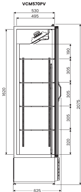
VISA COOLER RESFRIADOS 570L (INTERNO EM AÇO)
