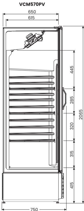
VISA COOLER RESFRIADOS 570L (INTERNO EM PSAl)
