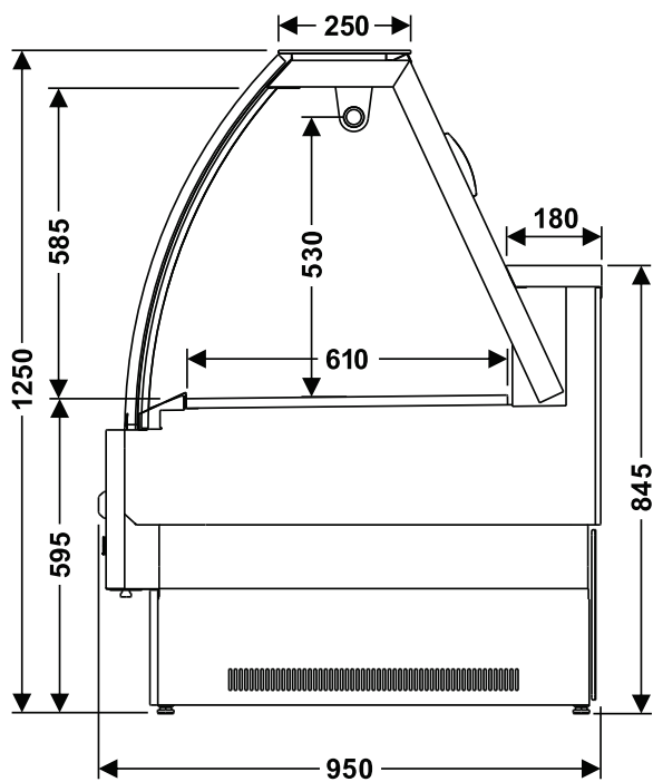
EXPOSITOR AÇOUGUE PREMIUM VIDRO CURVO GANCHEIRA
