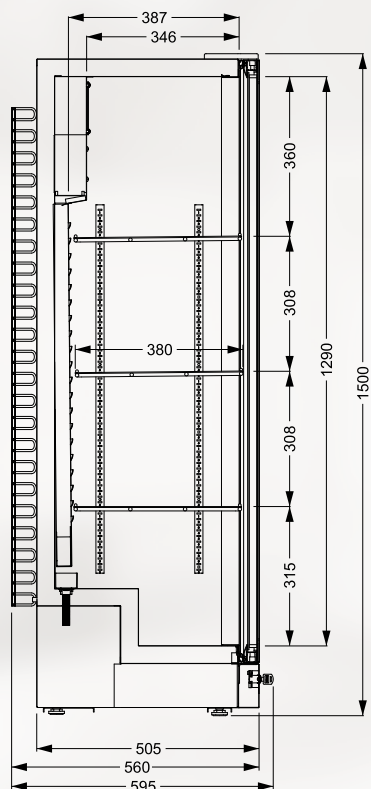
CERVEJEIRA HOME BEER 250 LITROS
