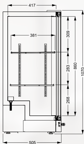
CERVEJEIRA HOME BEER 130 LITROS
