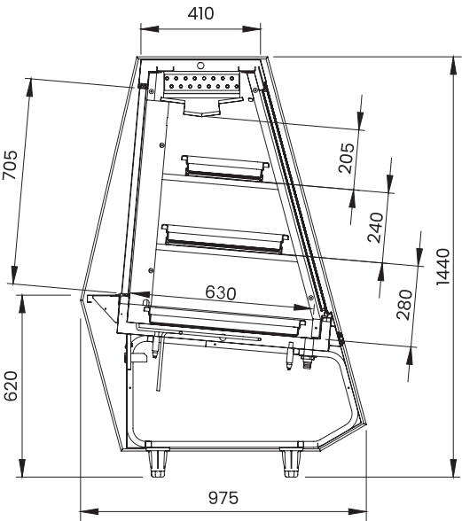
EXPOSITOR AÇOUGUE ATLANTIS PRATELEIRAS
