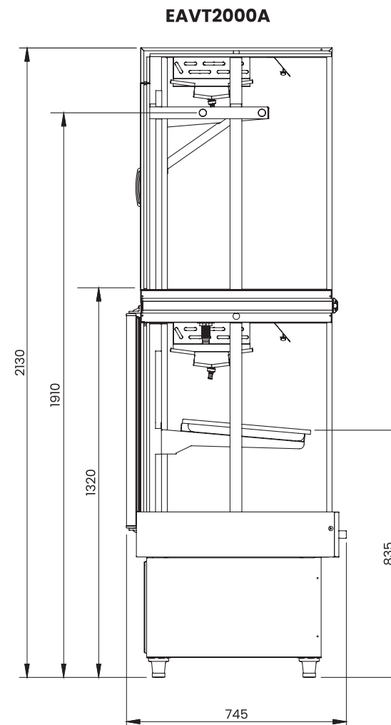
EXPOSITOR AÇOGUE VANGUARD TOP 2000 ALTO
