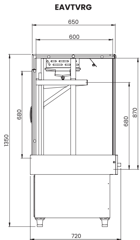
EXPOSITOR AÇOGUE VANGUARD TOP VIDRO RETO GANCHEIRA
