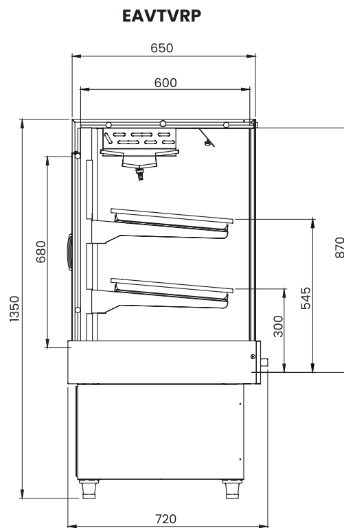
EXPOSITOR AÇOGUE VANGUARD TOP VIDRO RETO PRATELEIRA
