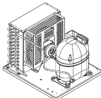
Figura 8: Figura Condensadora
