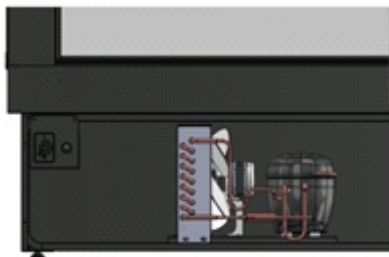
Figura 15: Unidade condensadora
