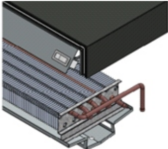
Figura 14: Evaporador
