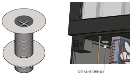
Figura 8: Detalhe do dreno de saída para água
