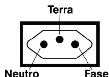
Figura 4: Tomada modelo nacional com fio terra
