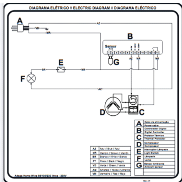
Figura 19: Diagrama eléctrico modelos AHW - 220V
