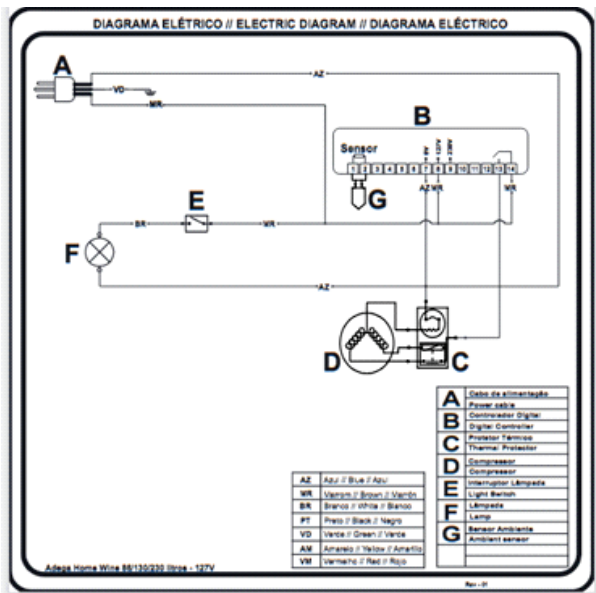
Figura 18: Diagrama eléctrico modelos AHW – 127V
