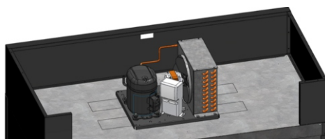
Figura 15: Acesso ao compressor modelo VCS 1900.
