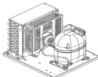
Figura 9: Unidade condensadora
