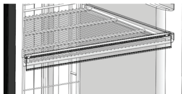
Figura 10: Montagem do perfil porta-etiquetas
