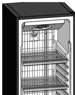
Figura 9: Colocação das prateleiras.
