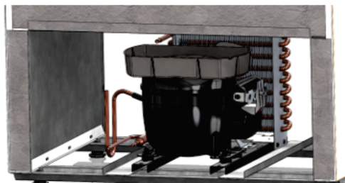
Figura 7: Compressor com bandeja coletora.
