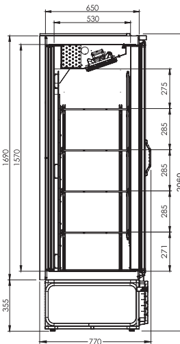
VISA COOLER CONGELADOS 1300
