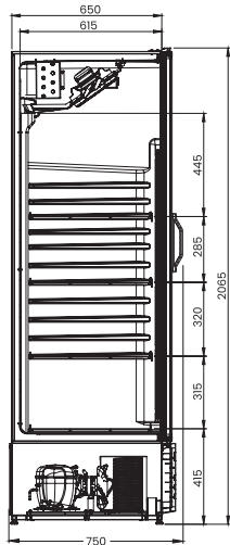
VISA COOLER RESFRIADOS 570
