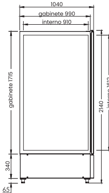
MINI CÂMARA GELO 1800L
