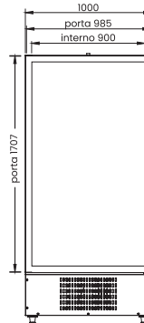
MINI CÂMARA GELO 1100L
