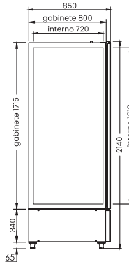
MINI CÂMARA GELO 1100L
