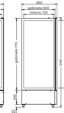
MINI CÂMARA GELO 700L
