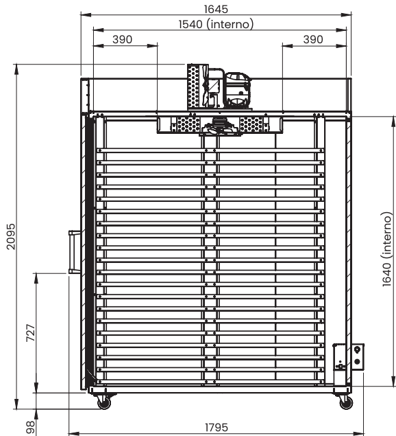
CÂMARA DE FERMENTAÇÃO 40 ESTEIRAS
