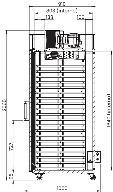
CÂMARA DE FERMENTAÇÃO 20 ESTEIRAS
