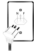
Figura 3: Plug modelo nacional com fio terra.
