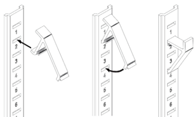
Figura 9: Fixação dos suportes das prateleiras.
