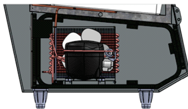
Figura 15: Unidade condensadora
