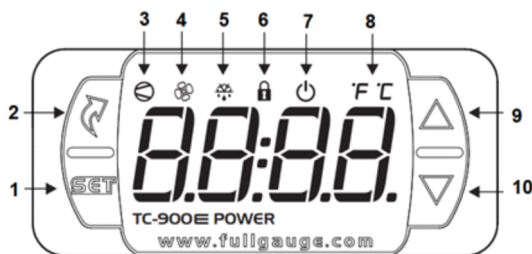
Figura 6: Controlador TC-900E POWER
