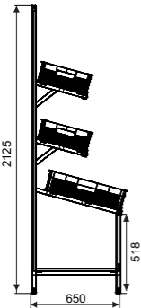
FRUTEIRA LATERAL PREMIUM 7 CAIXAS
