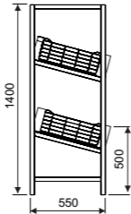
FRUTEIRA LATERAL PREMIUM 6 CAIXAS
