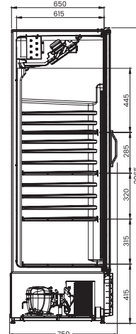
VISA COOLER MULTIUSO 570
