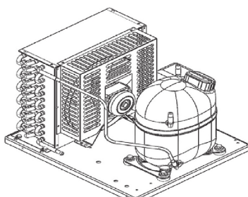
Figura 13: Unidade condensadora
