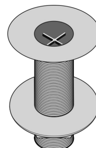
Figura 8: Detalhe do dreno de saída para água
